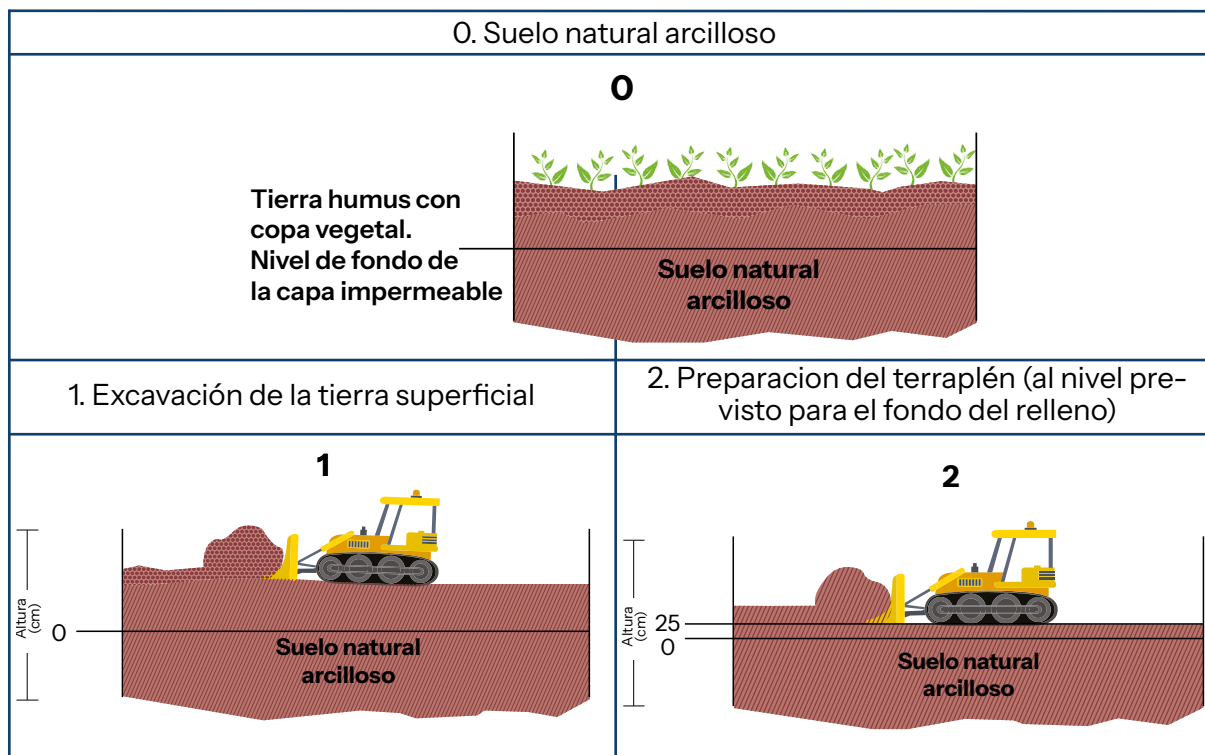
Figura 29. Construcción de capa base CON barrera natural.
