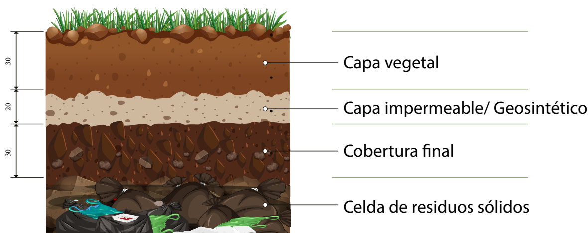
Figura 64. Capa final de la celda.
