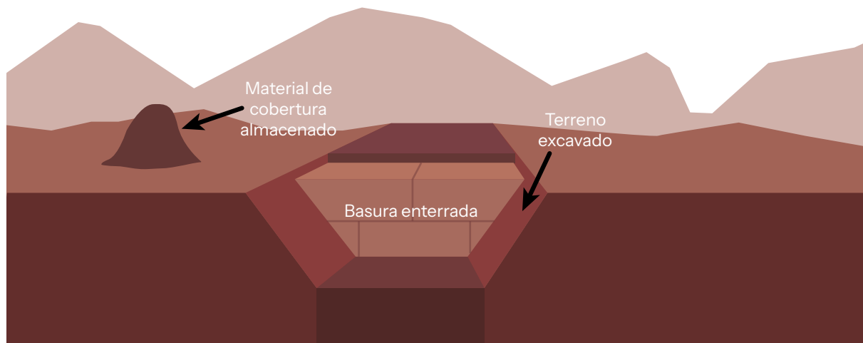
Figura 11. Método de trinchera.
