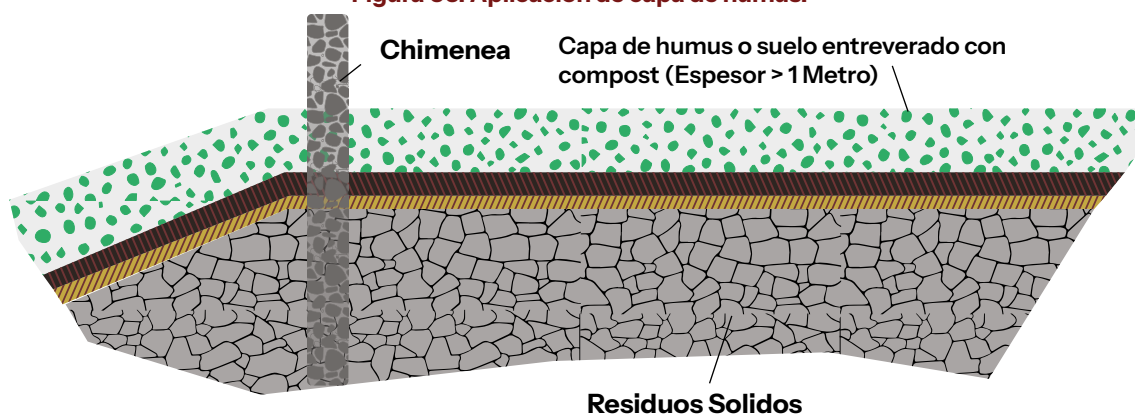
Figura 66. Aplicación de capa de humus.
