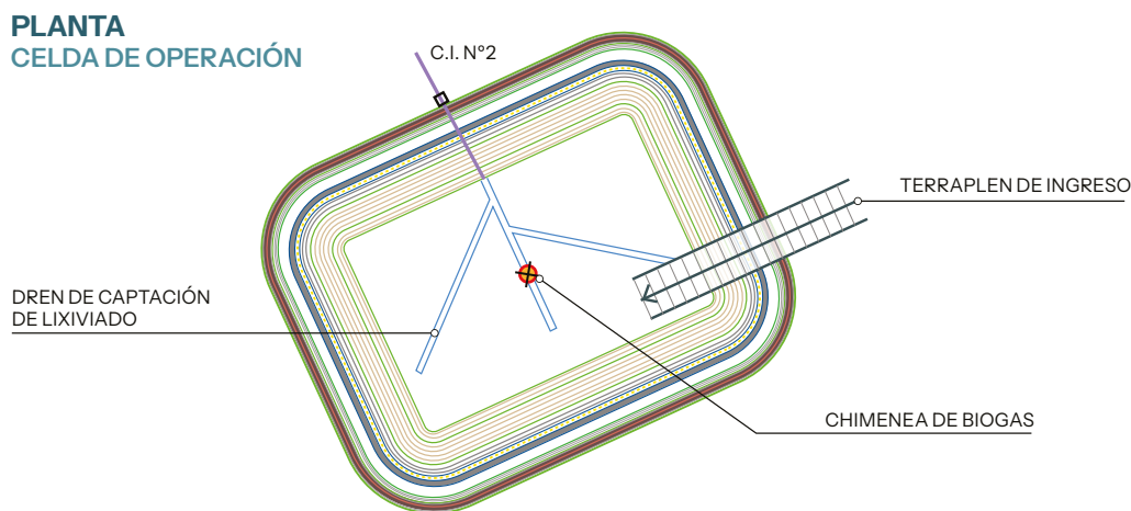
Figura 20. Distribución de sistema de drenaje de lixiviados.
