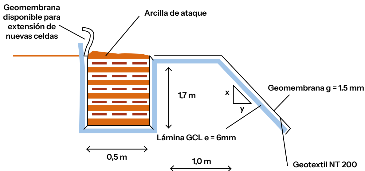
Figura 32. Anclaje geomembrana.
