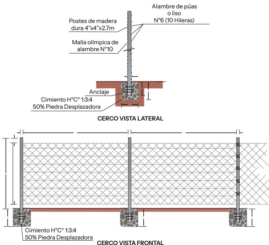
Figura 24. Cerco perimetral de rellenos sanitarios.
