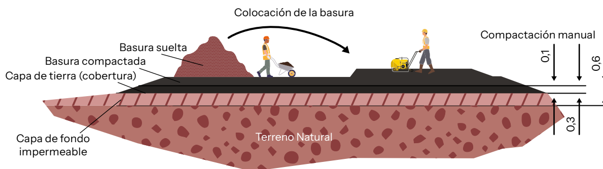
Figura 49. Colocación manual y compactación de residuos - Capas horizontales.
