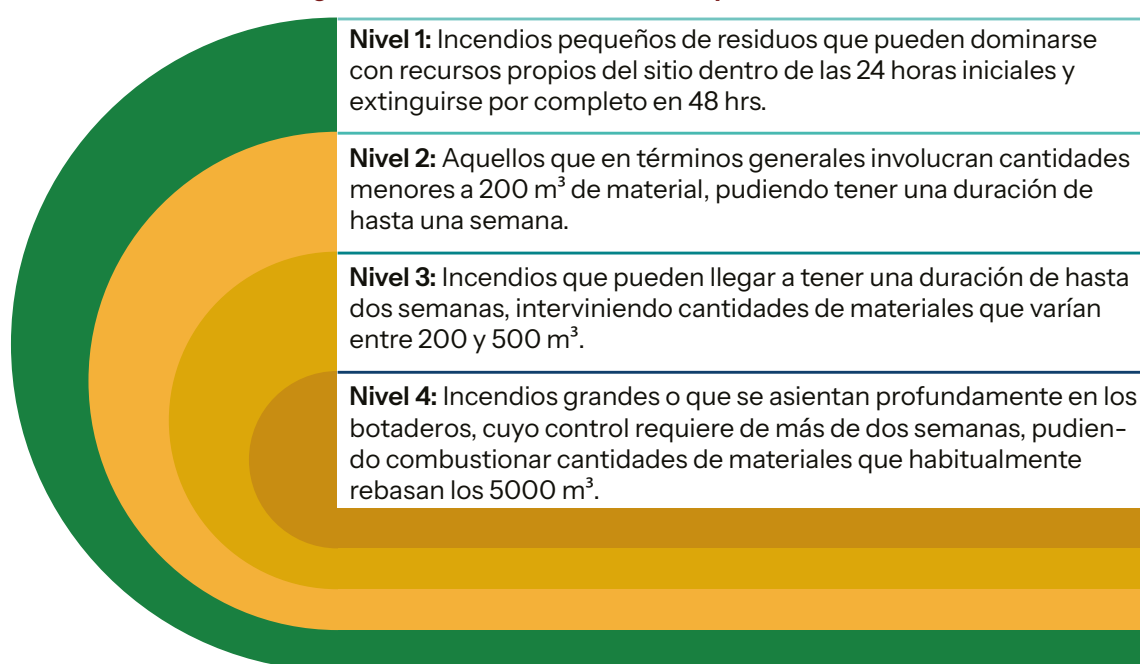
Figura 60. Niveles de incendios en disposición final.
