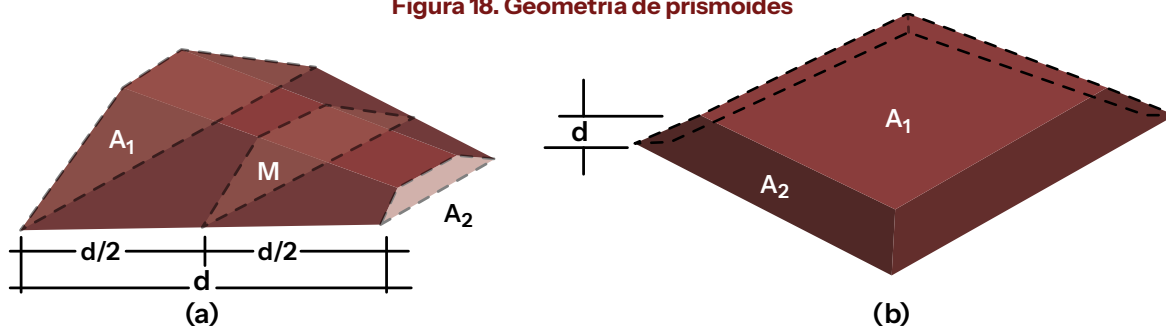
Figura 18. Geometría de prismoides
