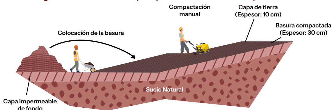
Figura 50. Colocación manual y compactación de los residuos - capas inclinadas.
