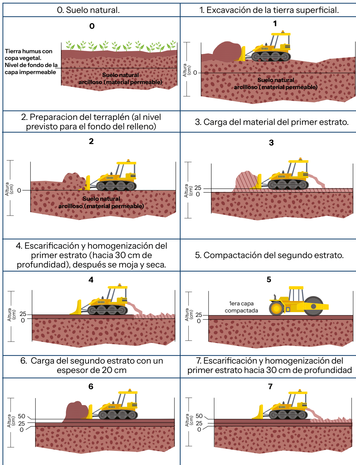
Figura 30. Construcción de capa base SIN barrera natural.
