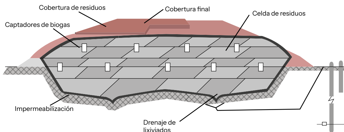
Figura 68. Esquema clausura del relleno sanitario.
