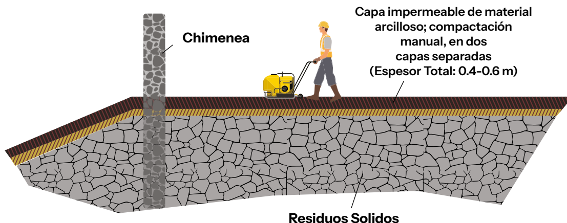
Figura 65. Construcción de capa impermeable.
