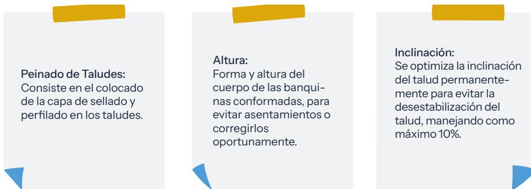
Figura 46. Recomendaciones en un crecimiento vertical de celdas.
