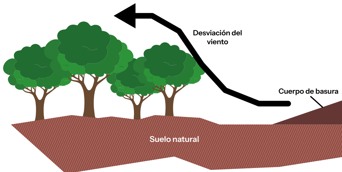
Figura 26. Detalle cerco vivo y franja de amortiguamiento.
