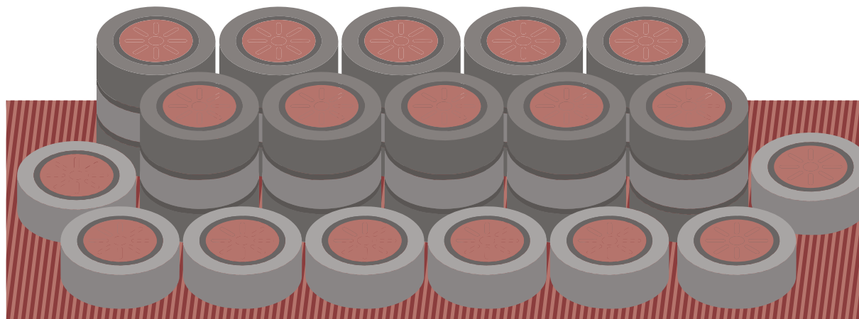
Figura 33. Muro de contención con llantas de desecho.
