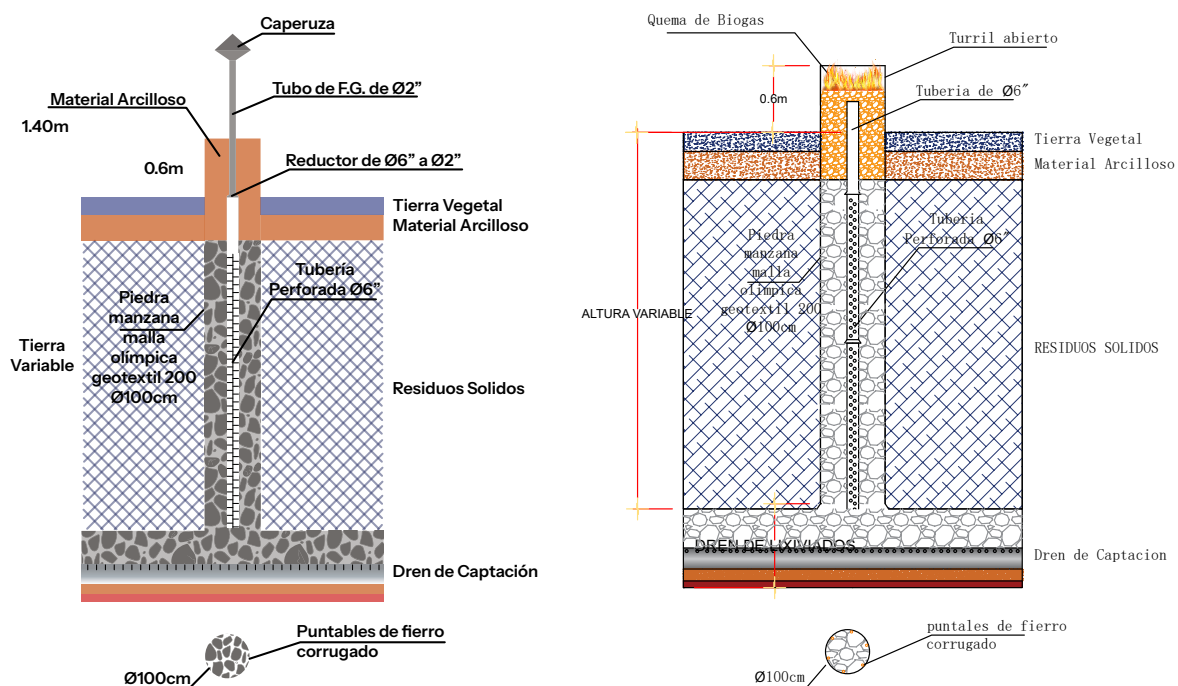
Figura 23. Construcción referencial de chimeneas.
