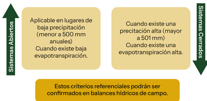
Figura 21. Criterios de precipitación y evapotranspiración para la selección de sistemas de almacenamiento de lixiviados.
