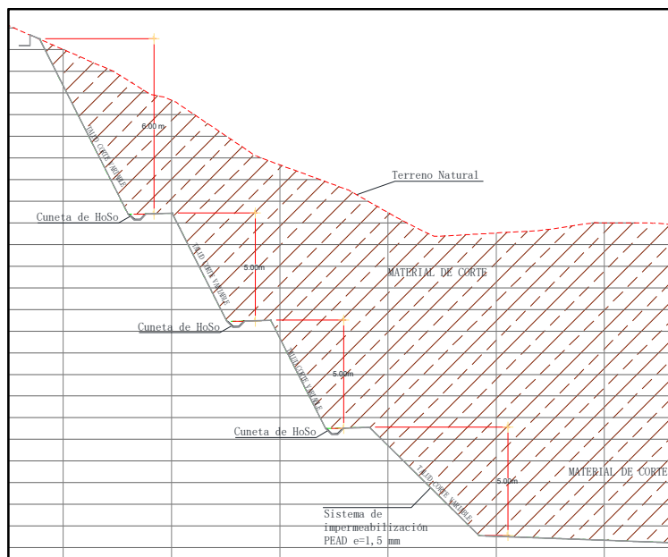
Figura 27. Imagen esquemática de corte talud-banquina para emplazamiento en terrenos ondulados.
