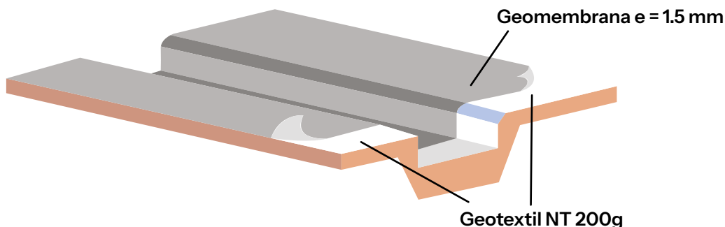
Figura 31. Sistema de impermeabilización sintética.
