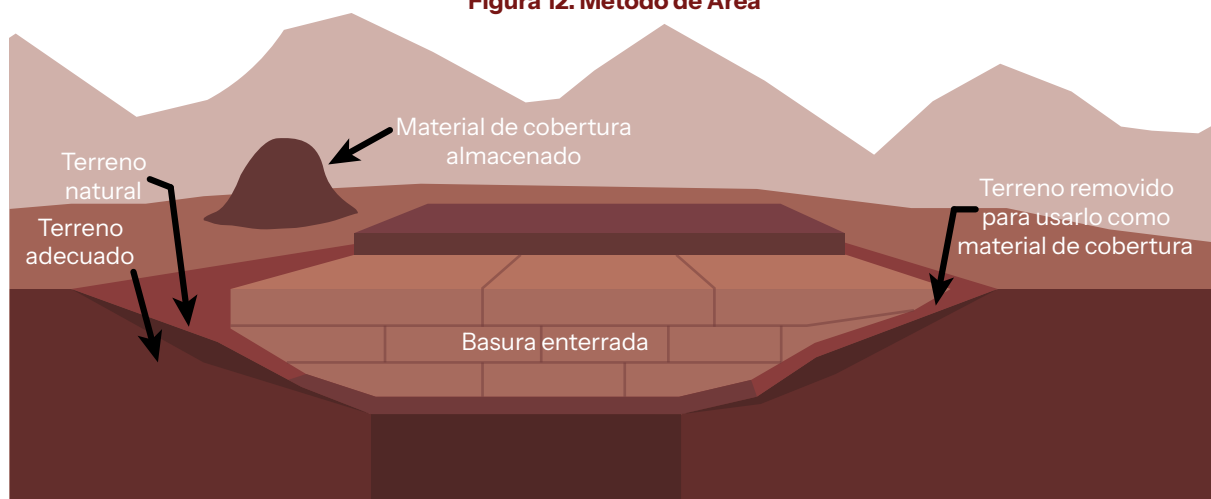
Figura 12. Método de Área
