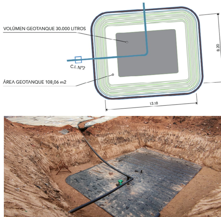
Figura 22. Sistema cerrado de almacenamiento de lixiviados, municipio de Cuevo
